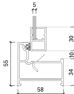
Dimenzije profila Mealon - nagibno odpiranje, E navadna zasteklitev
